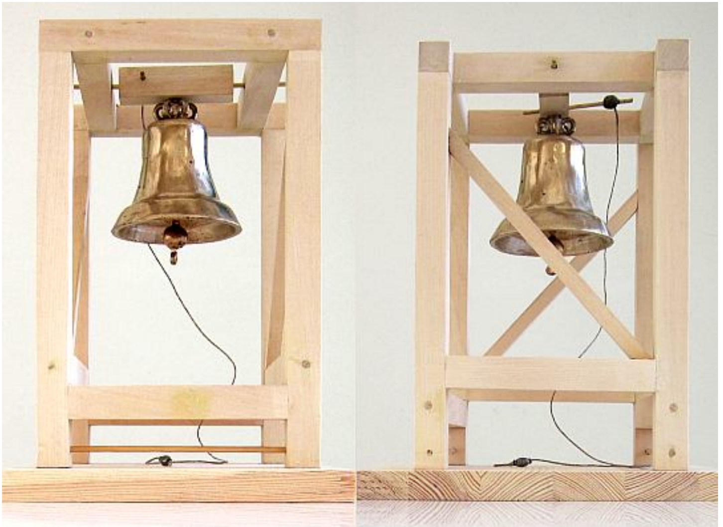
De hoogte van de toren is 27 cm, de breedte en de diepte 17 cm. De toren is gemaakt met lindenhout van 2x2 cm. De bodemplaat is 20x24 cm en 1,8 cm en gemaakt van verlijmd grenenhou.
